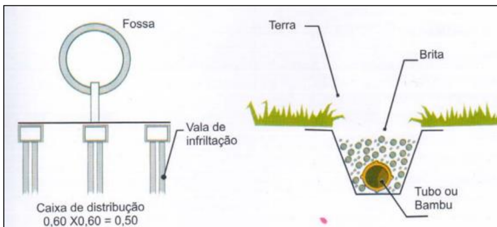
Figura 29 – Sistema de tratamento individual – Valas de Infiltração.
