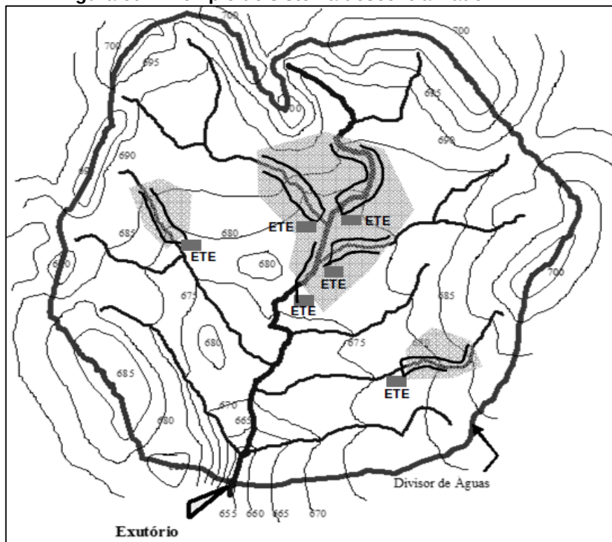
Figura 60 - Exemplo de sistema descentralizado.
