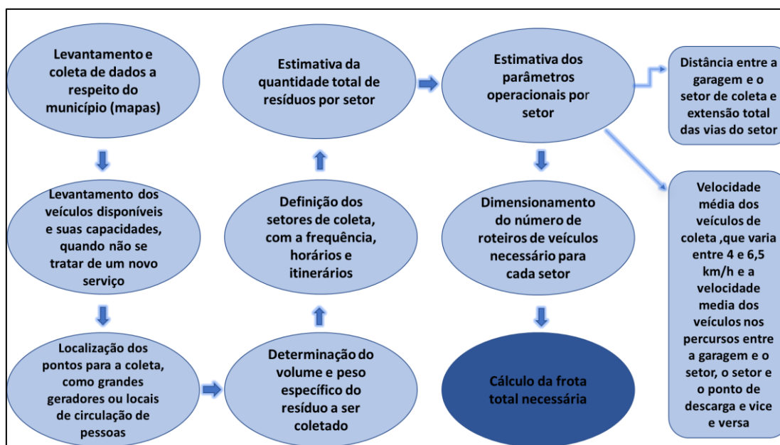
Figura 74 - Fluxograma das etapas mínimas do dimensionamento da coleta convencional.
