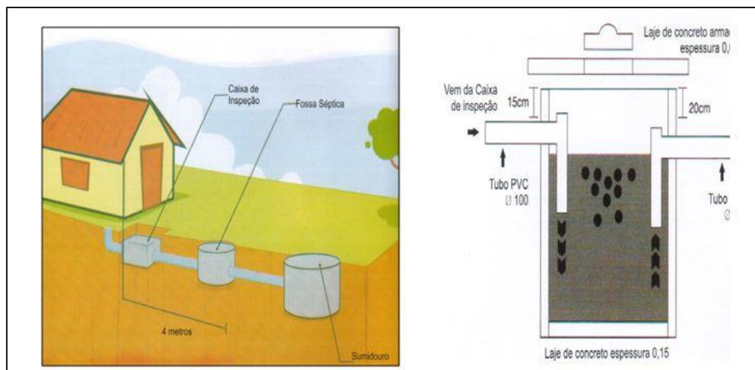
Figura 62 - Sistema Individual de Tratamento – Fossas Sépticas.
