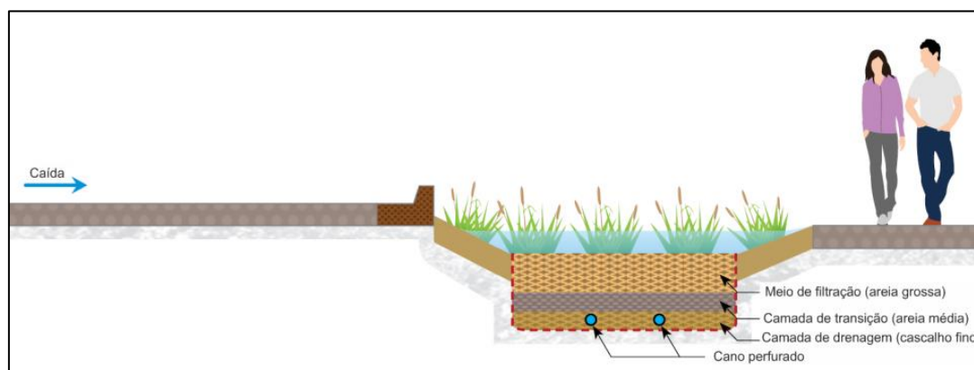
Figura 108 - Seção Típica de Valas Biorretenção.
