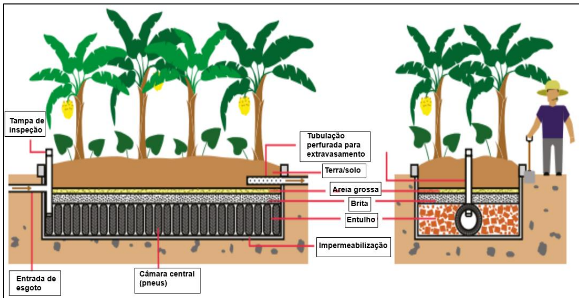
Figura 72 - Esquema de BET.
