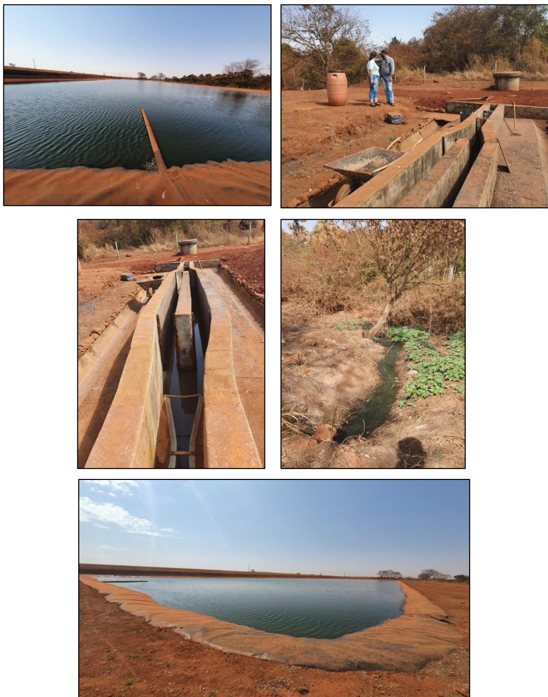
Figura 27- ETE de Água Comprida.
