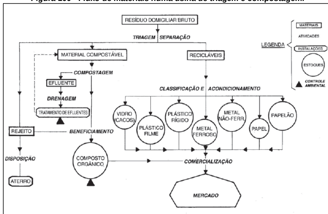
Figura 100 - Fluxo de materiais numa usina de triagem e compostagem.
