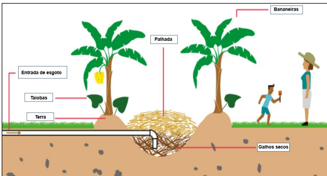
Figura 70 - Esquema de círculo de bananeira.
