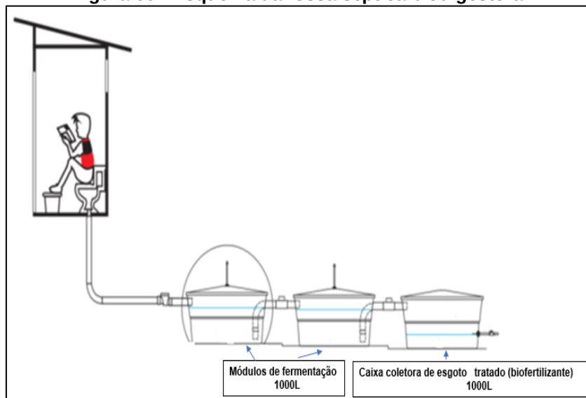
Figura 66 - Esquema da fossa séptica biodigestora.
