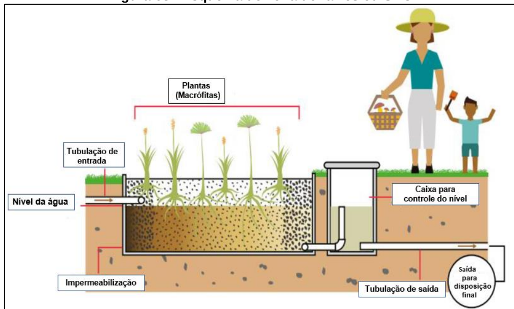
Figura 68 - Esquema de zona de raízes ou SAC.
