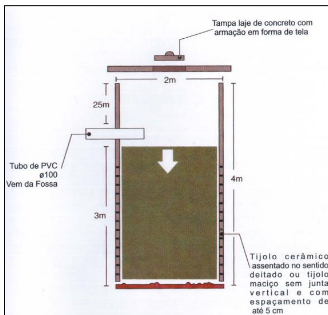
Figura 64 – Sistema individual de tratamento – Sumidouro.
