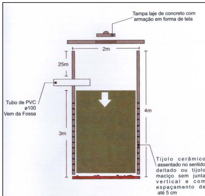
Figura 30 – Sistema individual de tratamento – Sumidouro.
