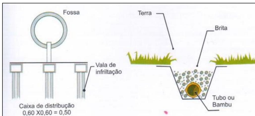
Figura 63 – Sistema de tratamento individual – Valas de Infiltração.
