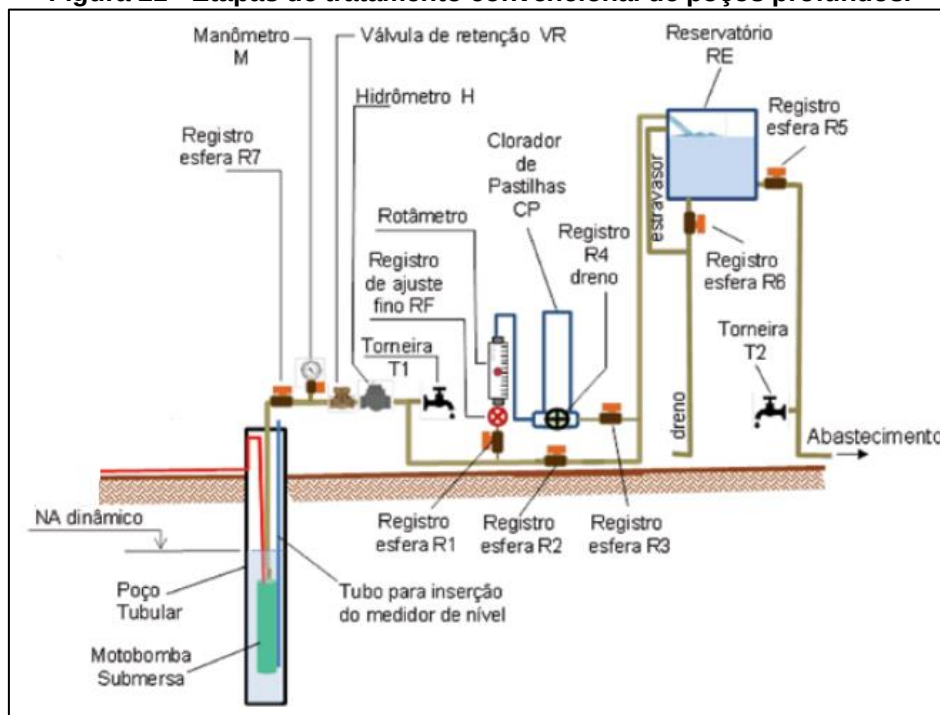
Figura 21 - Etapas de tratamento convencional de poços profundos.
