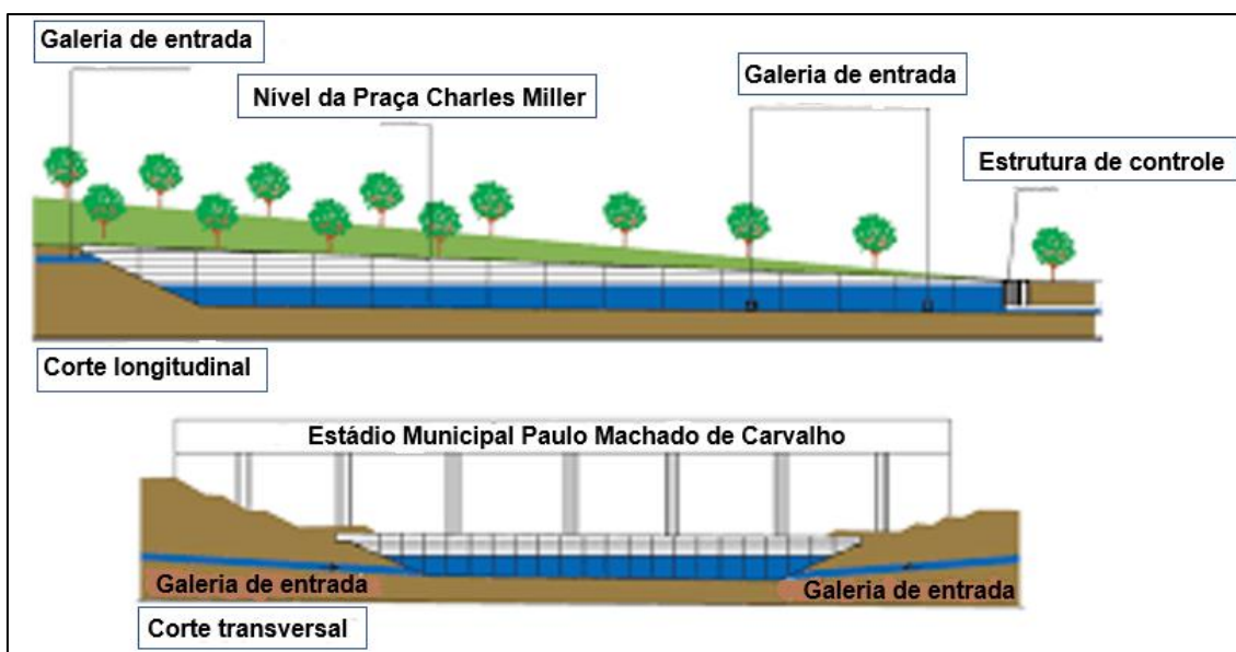
Figura 103 - Exemplo de Reservatório Subterrâneo com Recreação.
