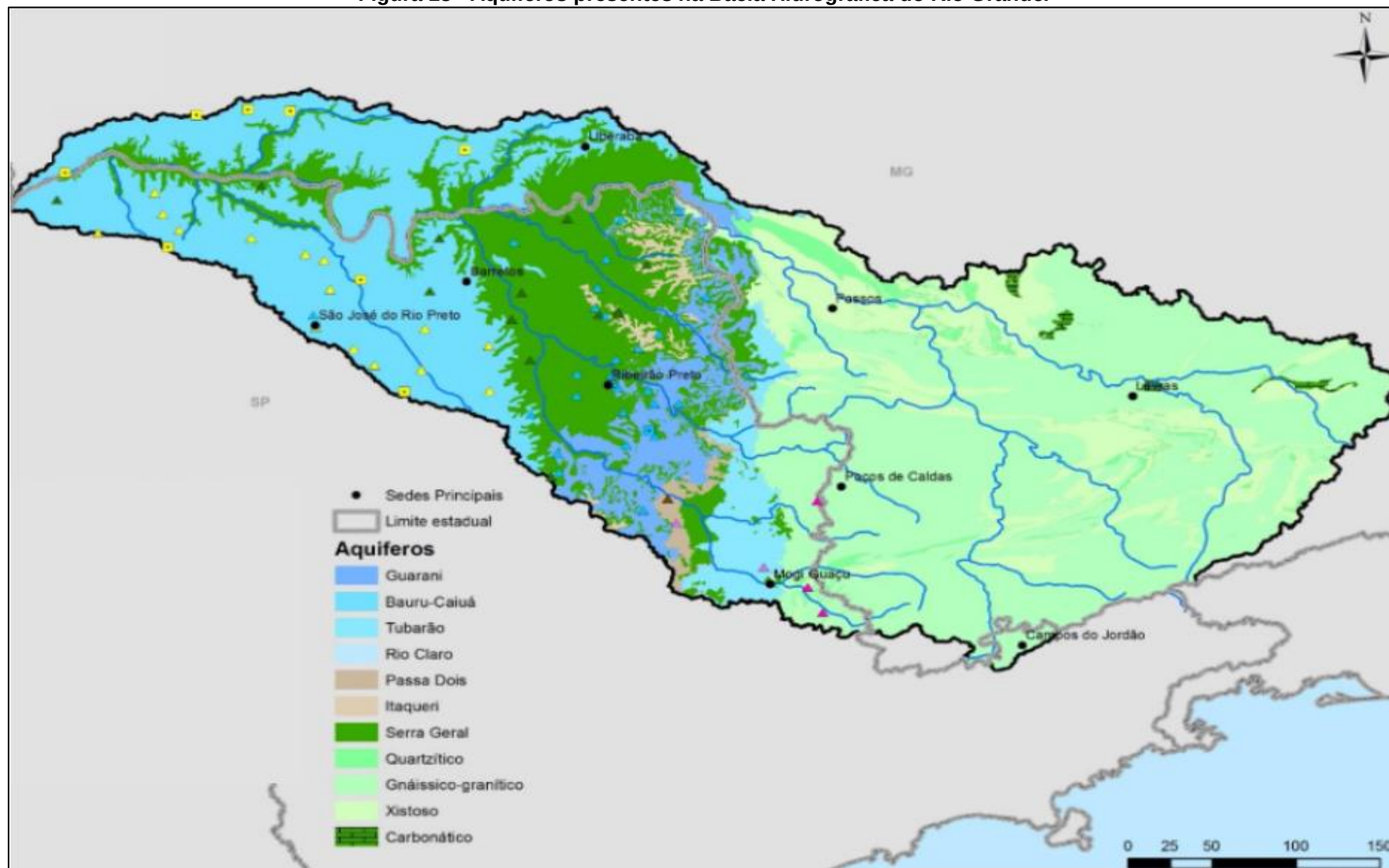
Figura 18 - Aquíferos presentes na Bacia Hidrográfica do Rio Grande.
