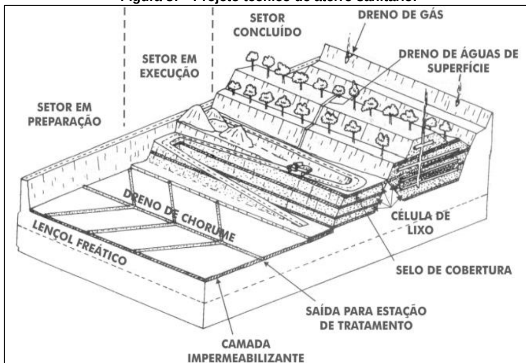
Figura 87 - Projeto técnico de aterro sanitário.
