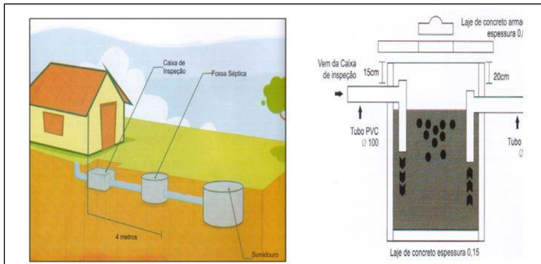
Figura 28 - Sistema Individual de Tratamento – Fossas Sépticas.
