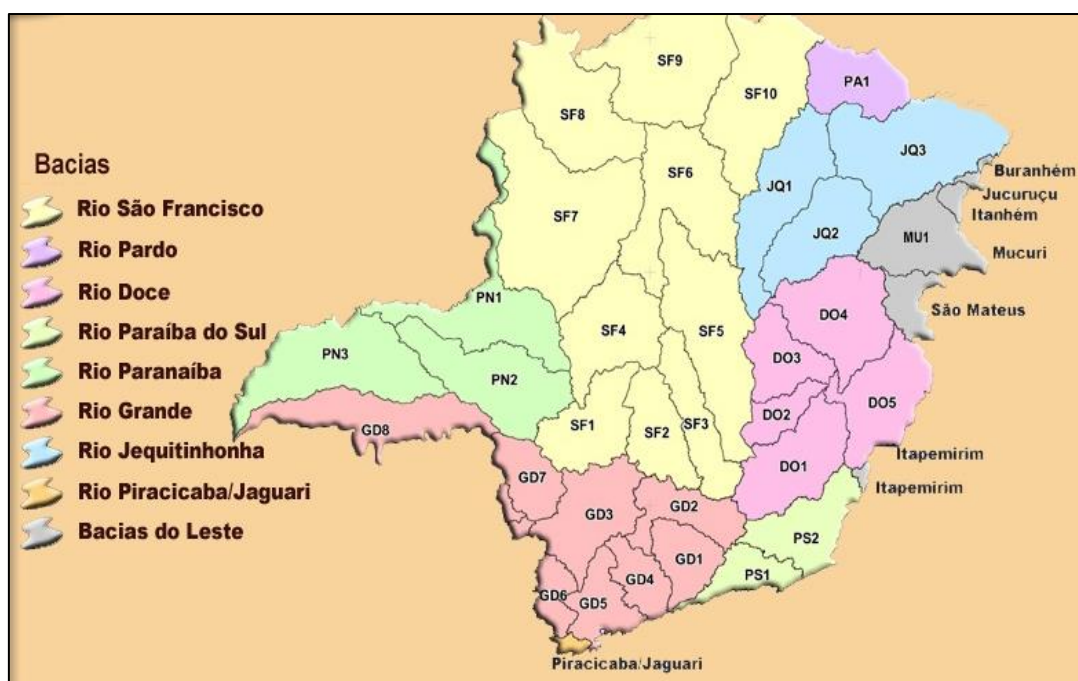
Figura 6 – Bacias Hidrográficas do Estado de Minas Gerais.
