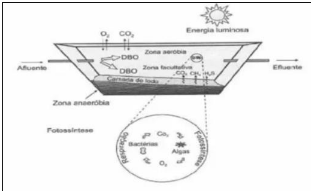
Figura 26 - Funcionamento da lagoa facultativa.
